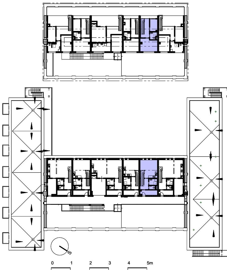
Schéma půdorys
